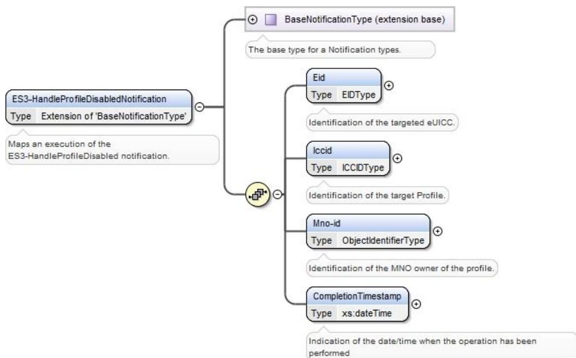
Figure 107: <rps:ES3-HandleProfileDisabledNotification>
