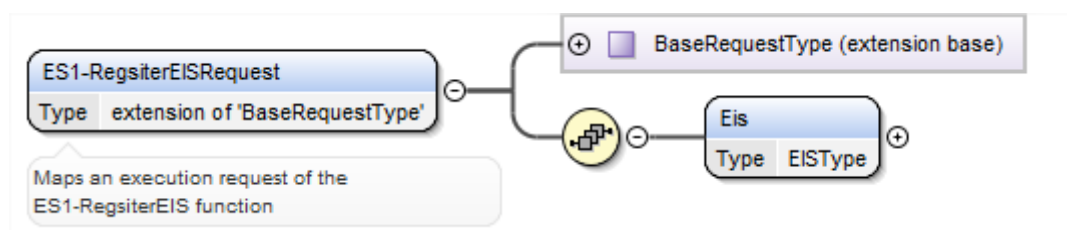
Figure 64 &lt;rps:RegisterEISRequest&gt;
