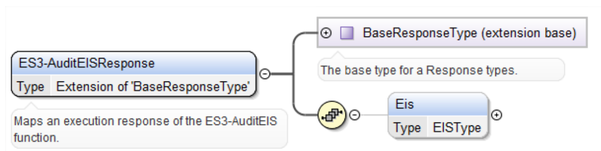
Figure 87 <rps:ES3-AuditEISResponse>
