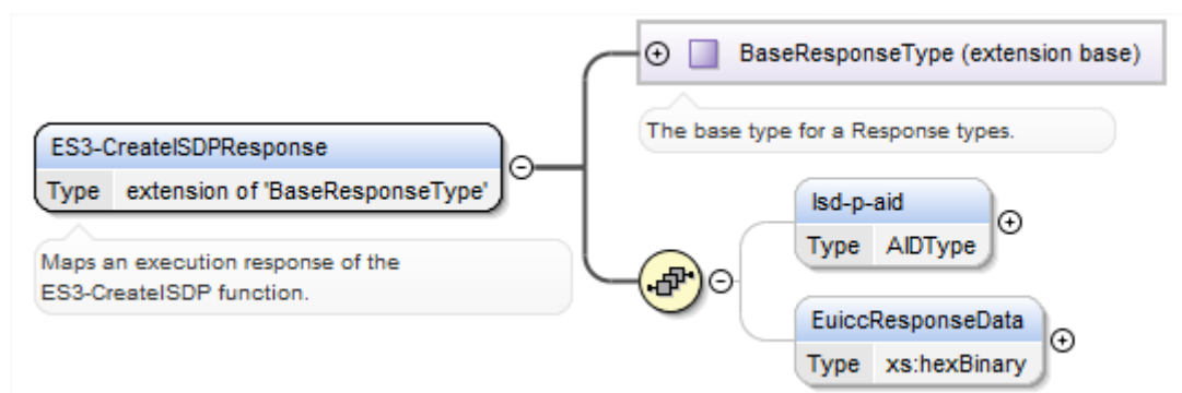
Figure 89 &lt;rps:ES3-CreateISDPResponse&gt;
