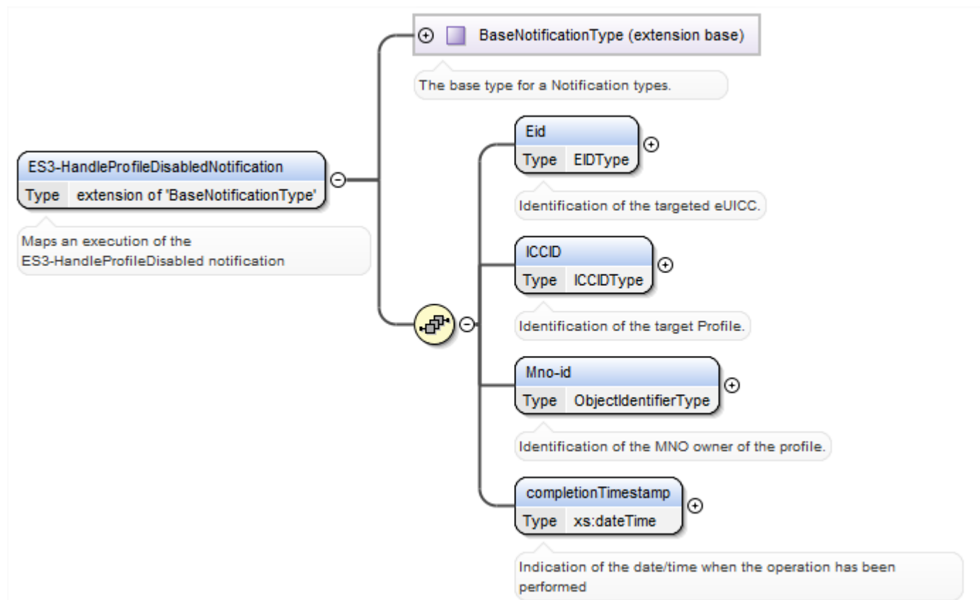
Figure 106 <rps:ES3-HandleProfileDisabledNotification>
