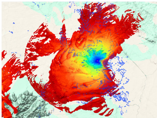
Couverture d'une cellule
