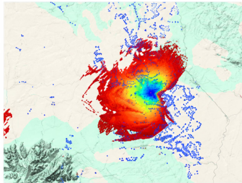
Couverture d'une cellule
