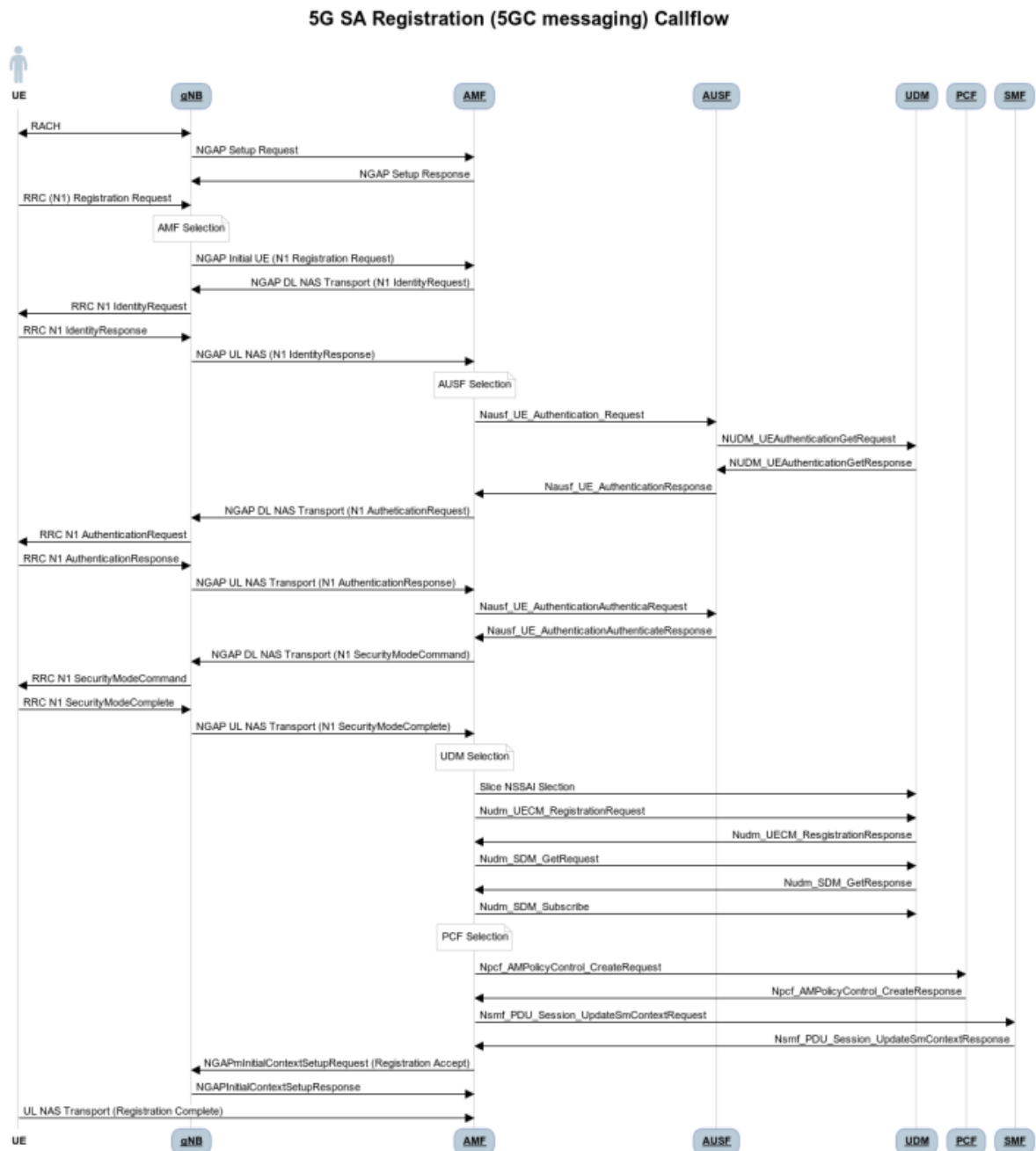
Figure 20 5G SA Registration
